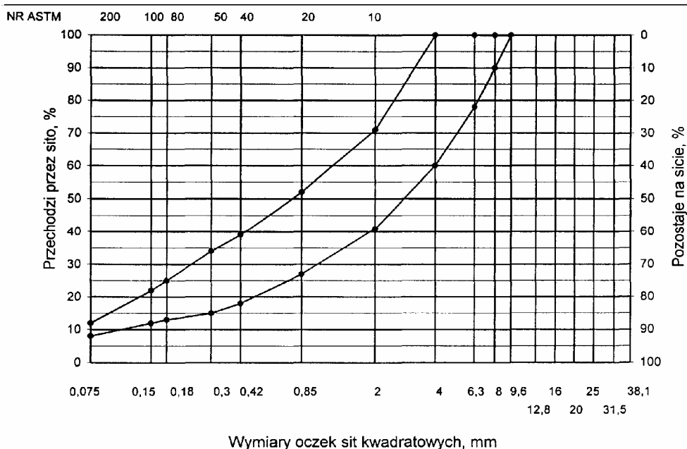
Rys. 3. Krzywe graniczne uziarnienia mieszanki mineralnej BA od 0 do 8mm, od 0 do 6,3 mm do warstwy wyrównawczej przy grubości minimum 2cm pod warstwę wzmacniającą z siatki stalowej
